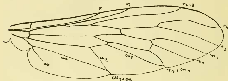
Fig. 2. Flügel 10 : 1.
